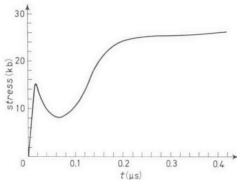
Fig. 21. - Precursor and shock in LiF. (J. ASAY, W.S.U.).
